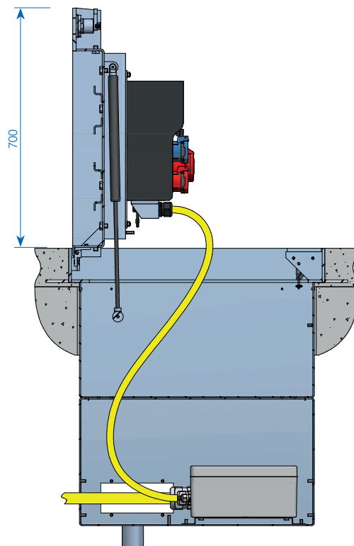
Seitenansicht offen
