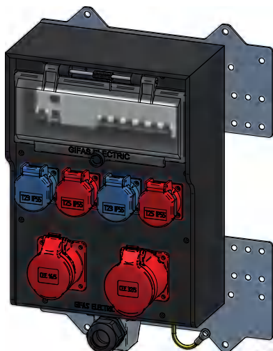
Stromverteiler
