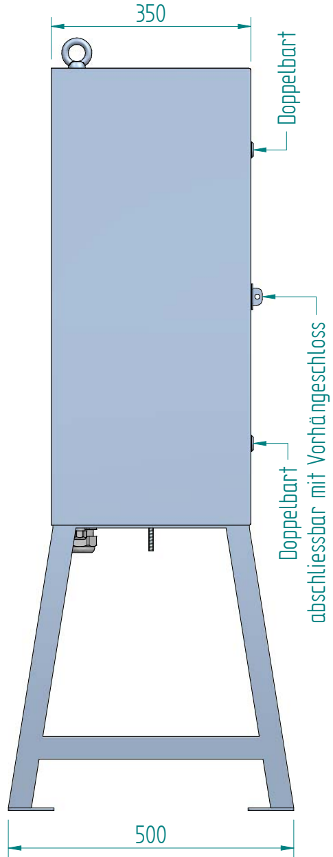
Schema Art.Nr. 231124
