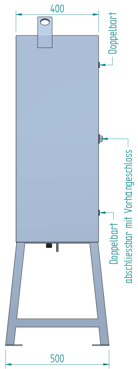
Schema Art.Nr. 231411
