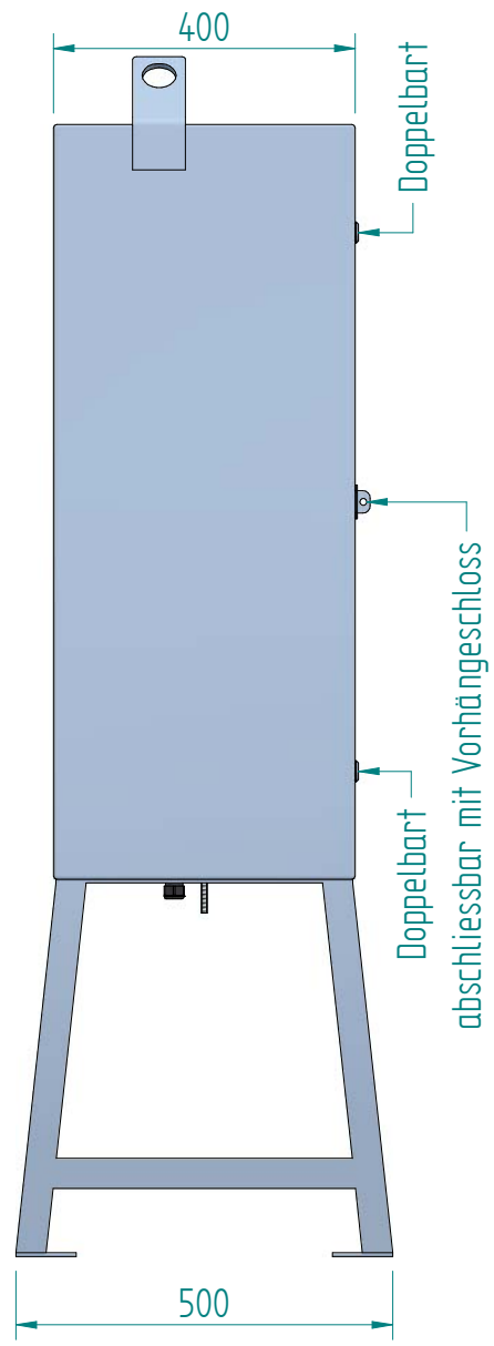
Schema Art.Nr. 231412
