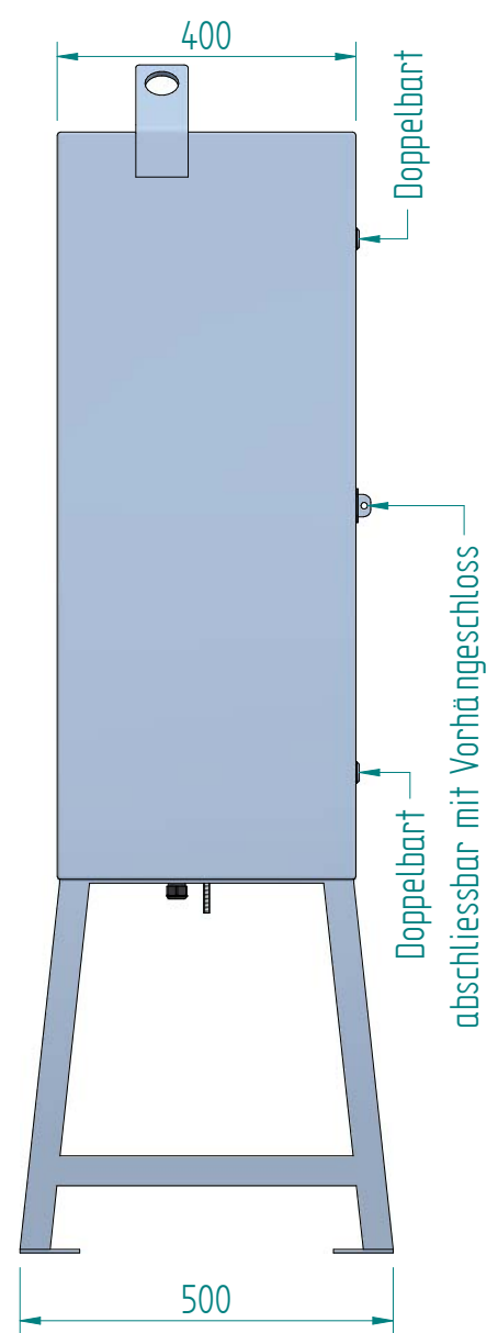
Schema Art.Nr. 231415
